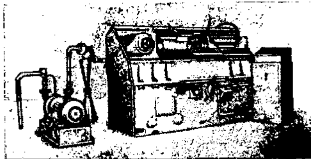
Рис. 4. Вихрекопировальный станок модели МА-459 для изготовления фасонных графитированных электродов.
