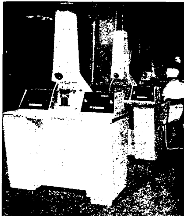
Рис. 1. Лазерные технологические установки К-3М на потоке.
