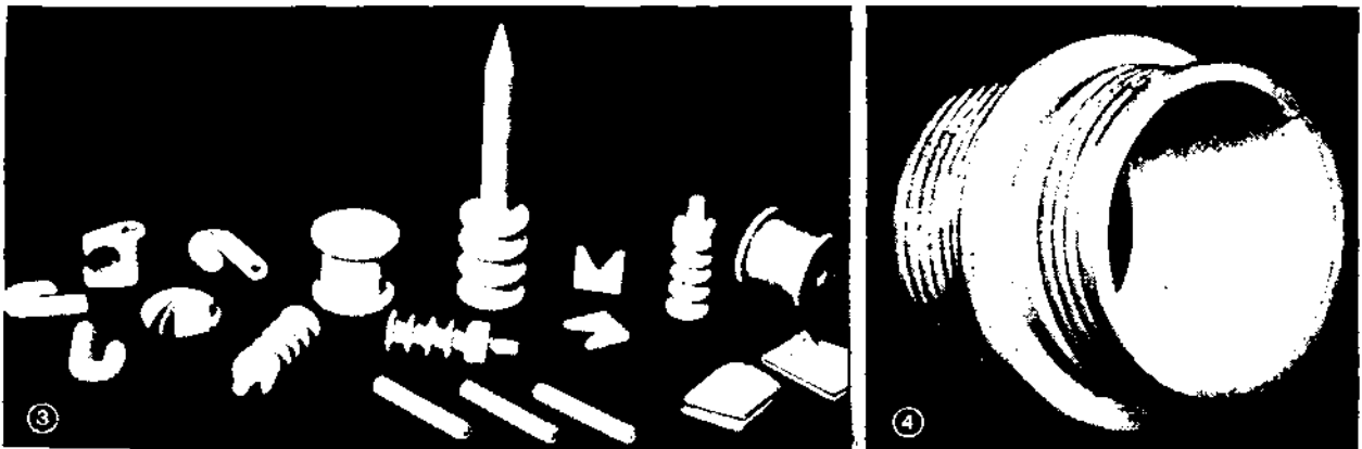
Рис. 3. Износоустойчивые детали на ситалла, применяемые при изготовлении химических волокон в текстильной промышленности. Рис. 4. Аппаратурные изоляторы из ситалла; наружный диаметр 500 мм, высота 500 мм.
