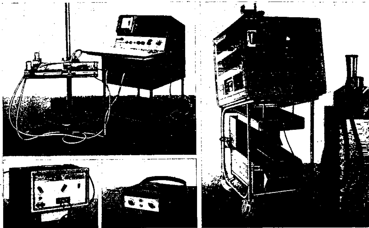
Рис. 1 (слева вверху). Радиотелеметрическая установка «Локация» с радиокапсулами. Рис. 2 (справа). Ультразвуковой диагностич. аппарат. Рис. 3 (слева внизу). Аппарат «Урат-1». Рис. 4 (в середине внизу). Портативный электрокардиостимулятор.
