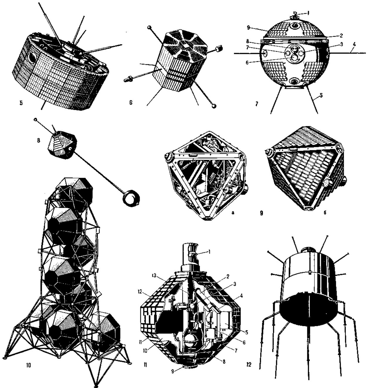
Рис. 5. Спутник ESSA-1. Рис. 6. Спутник OV-3. Рис. 7. Спутник «Эксплорер XXXII». 1 — масс-спектрометр нейтральных частиц; 2 — стыв днаща в обечайки корпуса; 3 — отверстие для шланга системы продувки; 4 — штырь электростатического аиода; 5 — штырь турникетной антенны; 6 — солнечные датчики и датчики направления на Луну; 7 — отверстие для шланга системы наддува; 8 — инфракрасный датчик аземного горизонта; 9 — солнечные элементы. Рис. 8. Спутник GGS. Рис. 9. Спутник ORS-2. а — до монтажа панелей с солнечными элементами; б — после монтажа панелей. Рис. 10. «Магазин» со спутниками для военной системы связи IUCSP. Рис. 11. Спутник для военной системы связи IUCSP. 1 — приемно-передающая антенна; 2 — фильтр в передающем устройстве; 3 — переключатель волновода; 4 — смеситель в передающем устройстве; 5 — усилитель промежуточной частоты; 6 — сопло для раскрутки спутника; 7 — умножитель частоты (в 11 раз); 8 — баллон со сжатым азотом; 9 — антенна телеметрического передатчика; 10 — панель для монтажа электронного оборудования; 11 — усилитель на ЛВВ; 12 — солнечные элементы; 13 — элемент конструкции. Рис. 12. Спутник ATS-1 (ATS-B). Рис. 13. Ракета «Аджена D» (GAT). 1 — основной двигатель; 2 — сопло системы ориентации; 3 — баллоны со сжатым азотом для сопел (2); 4 — вспомогательный двигатель; 5 — корпус ракеты; 6 — датчик горизонта; 7 — стыковочный насадок. Рис. 14. Аппарат ATDA в полете (снимок из кабели спутника «Джемини IX»). 1 — отсек батарей; 2 — отсеи двигателей системы ориентации; 3 — отсек электронного оборудования; 4 — держатель с ловушками; 5 — дипольная антенна радиолокационного ответчика; 6 — обтекатели, прикрывающие сварные болты; 7 — секции носового об-
