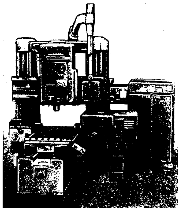
Рис. 1. Координатно-расточный станок модели 2B460.
