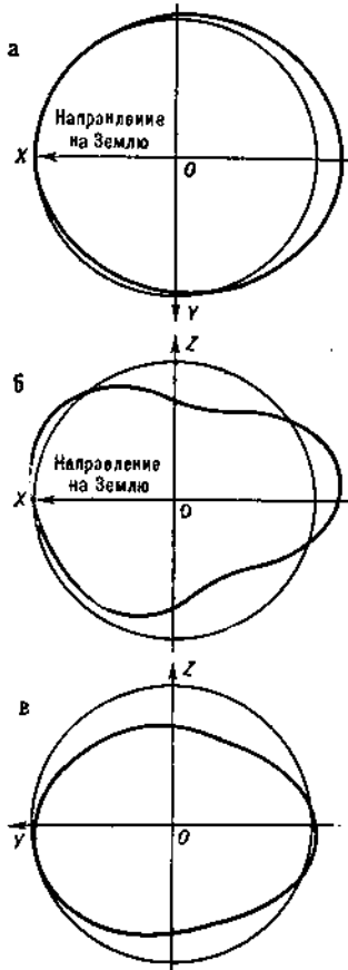
рис. 1. Сечения поверхности потенциала Луны экваториальной (а), меридиональной \lambda = 0^\circ (б) и меридиональной \lambda = 90^\circ (в) плоскостями.
