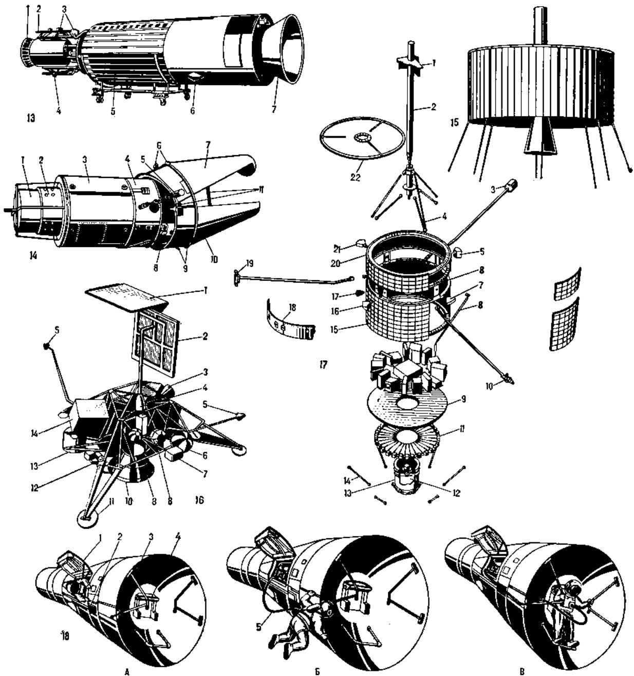
текатели; 8 — стыковочный насадок; 9 — крепления на бандаже (10); 10 — бандаж, стигивающий секции обтекателя; 11 — пружинные устройства для отбрасывания секций обтекателя. Рис. 15. Спутник «Лэни Бёрд I». Рис. 16. Космический аппарат «Сернейер I». 1 — панель с солнечными элементами; 2 — остроуправленная антенна; 3 — датчик звезды Канопус; 4 — панорамная телевизионная камера; 5 — всенаправленная антенна; 6 — баллон с гелием для подачи топлива в верхнерые двигатели; 7 — вспомогательная батарея; 8 — баллон со сжатым азотом для управляющих реактивных сопел системы ориентации; 9 — тормозной РДТТ; 10 — антенна радиолокатора АМР; 11 — опора посадочного шасси; 12 — верхнерый ЖРД; 13 — антенна доплеровского радиолокатора; 14 — контейнер с электронным оборудованием. Рис. 17. Космический аппарат «Пионер VII» (технологический разъем). 1 — антенна с низким коэффициентом усиления; 2 — антенна с высоким коэффициентом усиления; 3 — магнитометр; 4 — элемент крепления антенны 2; 5 — солнечный датчик; 6 — конструкция для крепления солнечных датчиков; 7 — солнечный датчик; 8 — антенна; 9 — монтажная полка; 10 — управляющее реактивное сопло; 11 — жалюзи; 12 — баллон со сжатым азотом; 13 — конструкция для крепления к ракете; 14 — элемент крепления; 15 — солнечные элементы; 16, 17, 21 — солнечные датчики; 18 — теплозащитный экран; 19 — устройство для демпфирования либрации; 20 — корпус аппарата; 22 — дноше корпуса (с теплозащитной). Рис. 18. Выход космонавта в открытый космос. А. Космонавт открывает люк и переносит в кабину держатель с ловушками. Б. Космонавт, кольнуясь поручнями, перемещается к вспомогательному отсеку спутника. В. Космонавт закрепляется в «седле» рацовой установки АМУ. 1 — крышка люка; 2 — держатель с ловушками; 3 — поручень; 4 — установка АМУ; 5 — фал.
