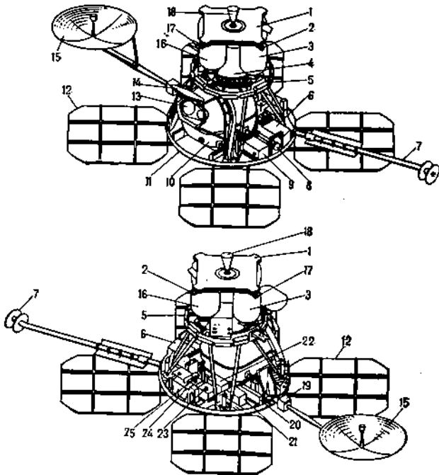
Рис. 4. Космический аппарат «Лунар орбитер 1». 1 — теплозащитный экран; 2 — солнечный датчик грубой ориентации; 3 — бак окислителя; 4 — несущая конструкция; 5 — детектор метеорных частиц; 6 — программно-временное устройство; 7 — всенаправленная антенна; 8 — датчик звезды Канопус; 9 — инерциальный блок; 10 — фотоустановка; 11 — платформа для монтажа оборудования; 12 — панель с солнечными элементами; 13 — объективы камер; 14 — теплоизолирующая крышка объективов; 15 — остроуправляемая антенна; 16 — бак горючего; 17 — управляющие реактивные сопла системы ориентации; 18 — бортовой ЖРД; 19 — привод антенны; 20 — усилитель на ЛБВ; 21 — декодирующее устройство; 22 — кодирующее устройство и мультиплексер; 23 — аккумуляторная батарея; 24 — передатчик; 25 — оборудование энергетической системы.
